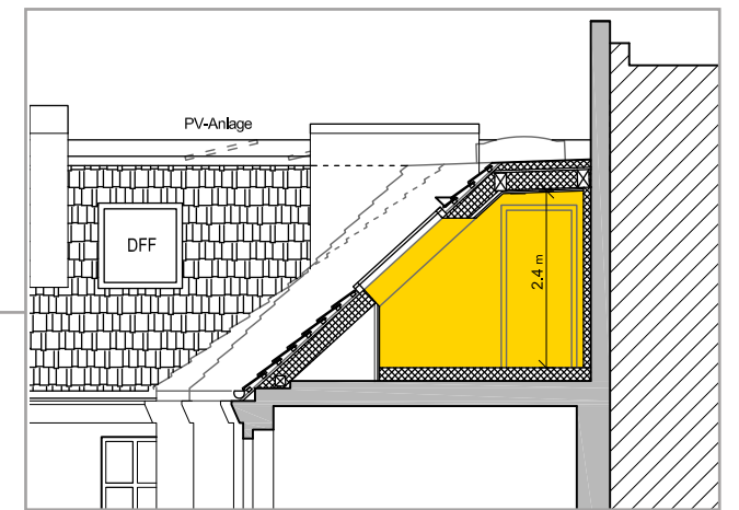
Schnitt Seitenflügel
